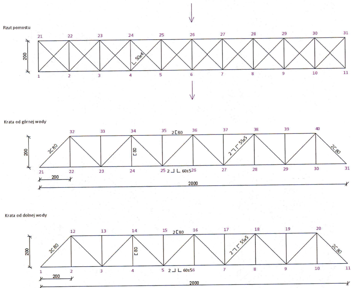
Rys. 1: Oznaczenia węzłów na schemacie elementów kładki
